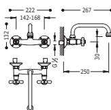
Gruppo lavello parete Distanza da parete di 250 mm. Wall sink mixer Distance from wall 250 mm. Nástěnný dřezový kuchyňský set vzdálenost od zdi 250 mm
