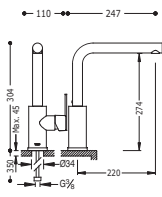
Monocomando lavello verticale Single lever single hole sink mixer Jednopáková dřevěová kuchyňská baterie
