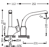
Monocomando lavello verticale Single lever single hole sink mixer Jednopáková dřezová baterie svislá
