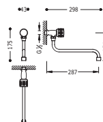
Monocomando lavello verticale Single hole sink mixer Otočná dřezová baterie 1/2"
