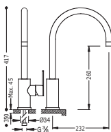
Monocomando lavello verticale Single lever single hole sink mixer Jednopáková dřevěová kuchyňská baterie
