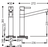
Monocomando lavello verticale canna lunga Single lever single hole sink mixer tube spout Jednopáková dřevěová kuchyňská baterie dlouhé ramínko
