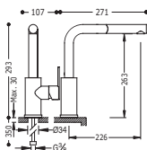
Monocomandoavello verticale estraibile
