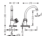
Monocomando lavello verticale Single lever single hole sink mixer Dřezová baterie, boční páka
