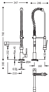
Monocomando lavello verticale Single lever single hole sink mixer Jednopáková dřezová kuchyňská baterie
