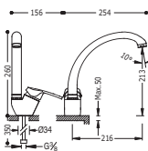
Monocomando lavello verticale Single lever single hole sink mixer Jednopáková dřezová baterie svíslá
