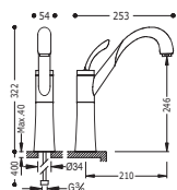
Monocomando lavello verticale Single lever single hole sink mixer Jednopáková dřezová baterie vislá
