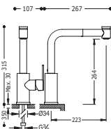
Monocomandoavello verticale estraibile (2 funzioni)
