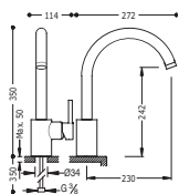
Monocomando lavello verticale Single lever single hole sink mixer Jednopáková dřevěová kuchyňská baterie
