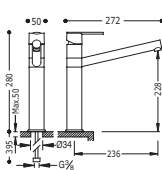
Monocomando lavello verticale canna lunga Single lever single hole sink mixer tube spout Jednopáková dřevěová kuchyňská baterie dlouhé ramínko
