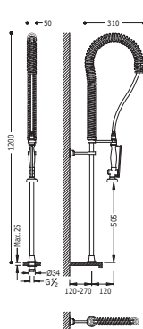
Monocomando lavello verticale Single lever single hole sink mixer Dřezová kuchyňská baterie
