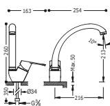
Monocomando lavello verticale Single lever single hole sink mixer Jednopáková dřezová kuchyňská baterie
