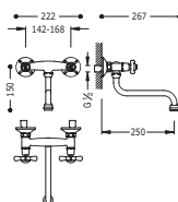
Gruppo lavello parete Distanza da parete di 250 mm. Wall sink mixer Distance from wall 250 mm. Nástěnný dřezový kuchyňský set vzdálenost od zdi 250 mm
