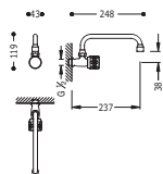
Monocomandoavello verticale Single hole sink mixer Otočná dřezová baterie 1/2"
